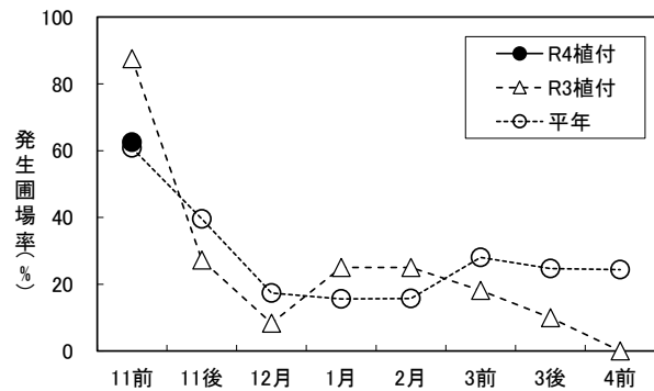
図2 きゅうりのコナジラミ類 発生圃場率の推移
