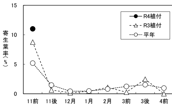
図1 きゅうりのコナジラミ類 寄生葉率の推移
