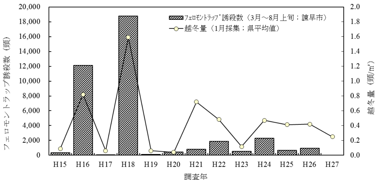
図1 チャバネアオカメムシのフェロモントラップ誘殺数と越冬量との関係
