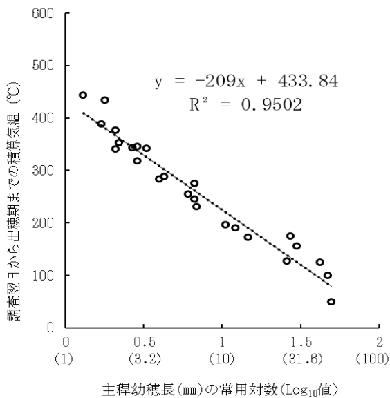
図 1 主稈幼穂長の常用対数と調査翌日から出穂期までの積算気温（2013年～2019年播）
