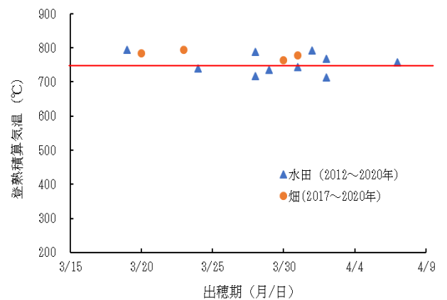
図 2 出穂期と出穂期翌日から成熟期までの登熟積算日数（2011年～2019年播）
