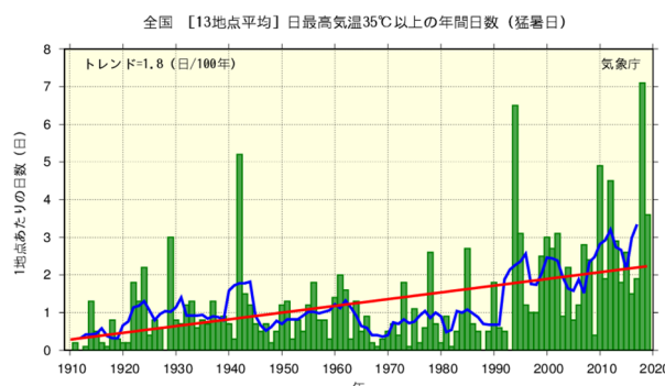
18 図211 日最高気温30 以上(真夏日、左図)、35 以上(猛暑日、右図)の年 19 間日数の経年変化(統計期間1910~2019年) 20 (出典:気候変動監視レポート2019)
