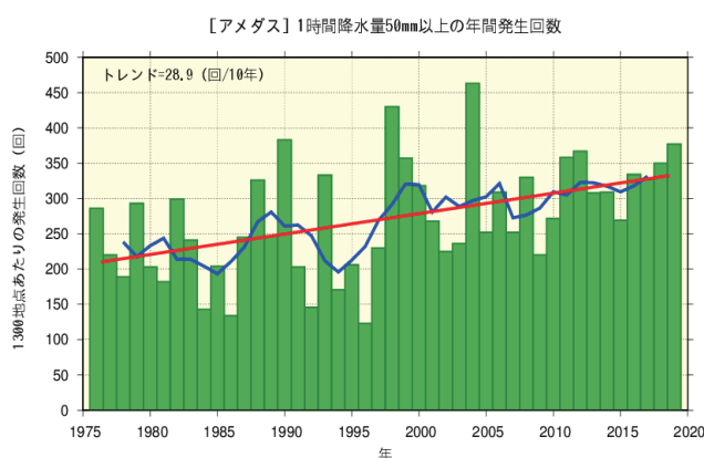
14 図210 日本の1時間降水量50mm以上の年間 15 発生回数の経年変化(1976~2019年) 16 (出典:気候変動監視レポート2019)
