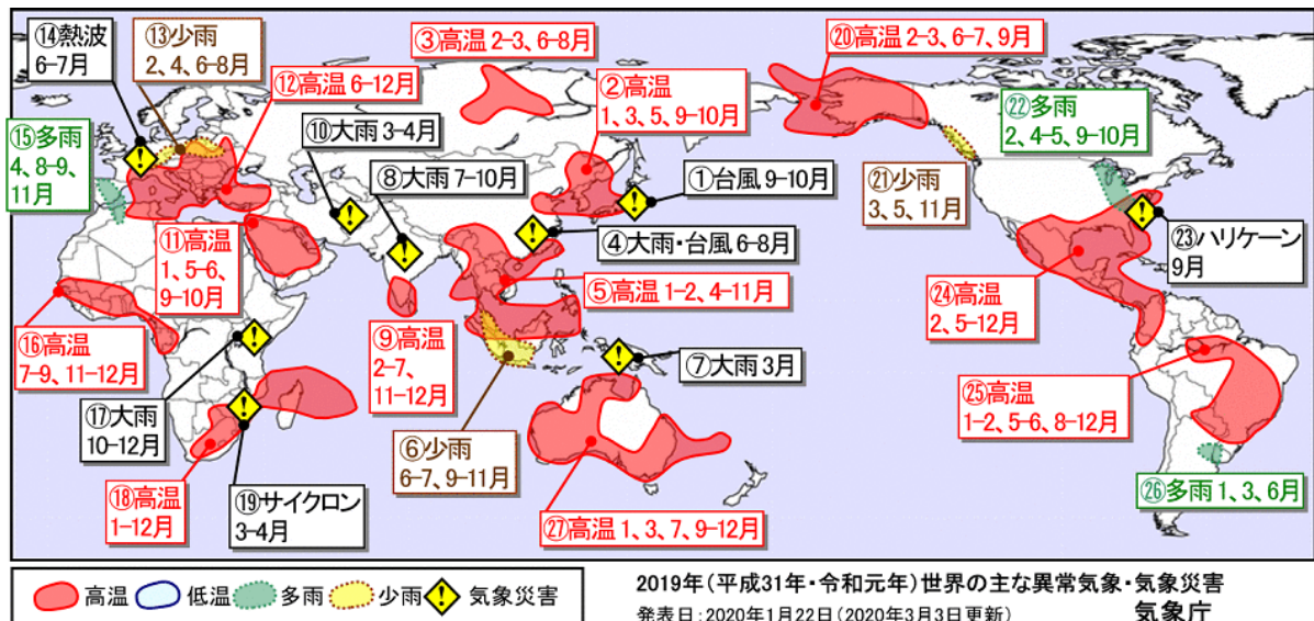
21 図2-3 世界の主な異常気象・気象災害の分布図 22 (出典: 気候変動監視レポート 2019)
