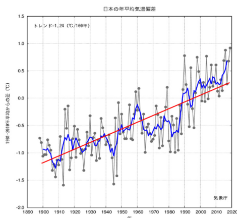
12 図29 日本の年平均気温偏差の経年変化 13 (出典:気候変動監視レポート2019)
