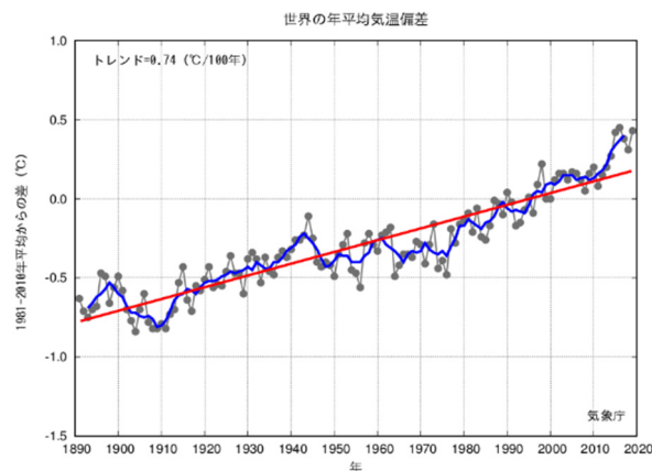
3 図2-4 世界の年平均気温の変化（出典：気候変動監視レポート2019）
