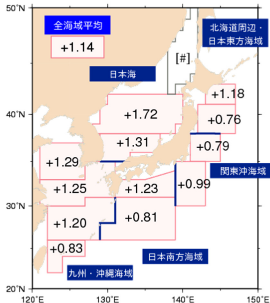
図 2 13 日本近海の海域平均海面水温 (年平均) の変化傾向 ( /100 年) (出典：気候変動監視レポート 2019)
