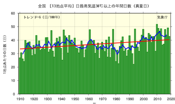
18 図211 日最高気温30 以上(真夏日、左図)、35 以上(猛暑日、右図)の年 19 間日数の経年変化(統計期間1910~2019年) 20 (出典:気候変動監視レポート2019)
