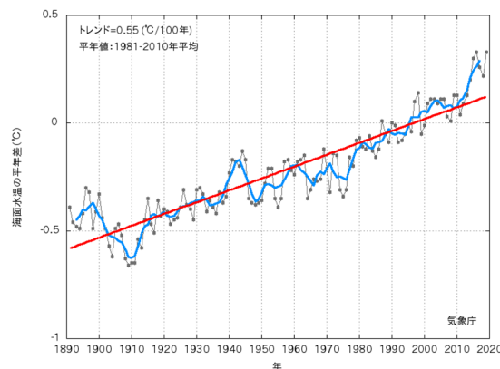
9 図2-5 世界全体の年平均海面水温平年差の経年変化(1891~2019年) 10 (出典：気候変動監視レポート2019)
