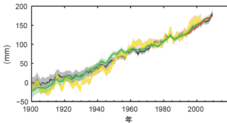
図 2-6 世界の平均海面水位の変化 (出典：IPCC 第 5 次評価報告書 第 1 作業部会報告書「政策決定者向け要約」)
