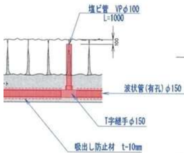
（護岸構造図、上から見た図）
