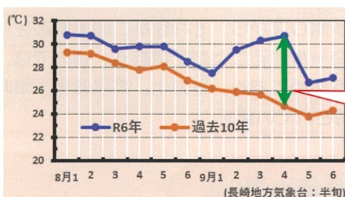
令和6年8～9月の半旬別平均気温
