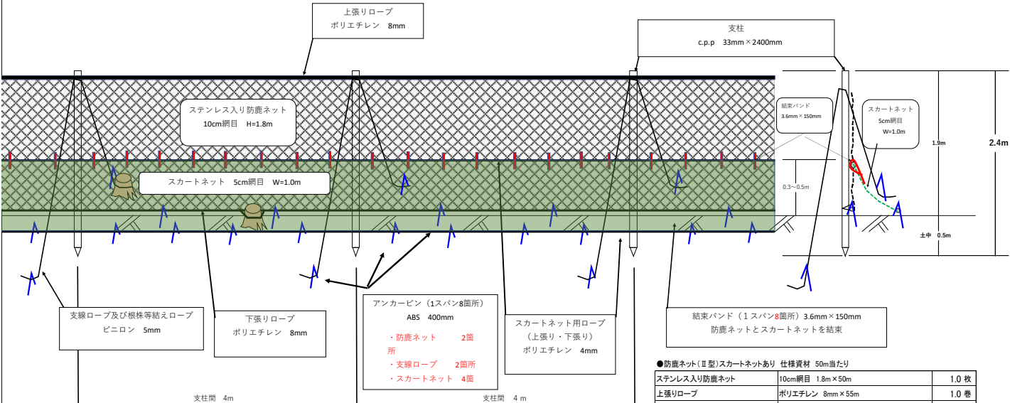
防鹿ネット（Ⅱ型） 後付けネット型 標準図
