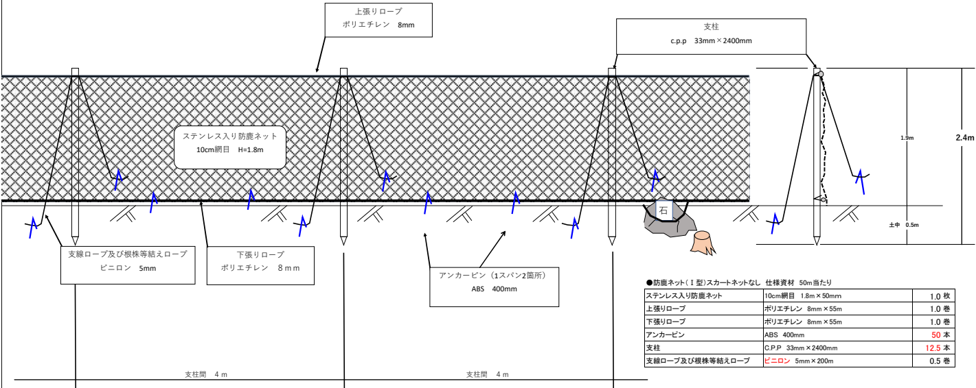
防鹿ネット（Ⅰ型） 後付ネット無型 標準図
