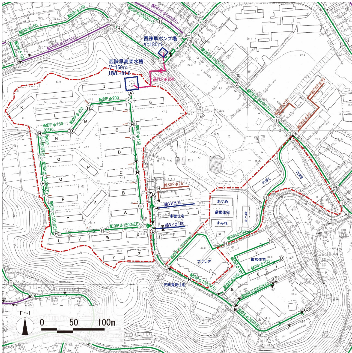
上水管路図（資料：諫早市水道課 提供資料）
